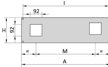
Панели/Двери модульные для измерительных приборов OptiBox M с 2 вырезами 92х92 мм
