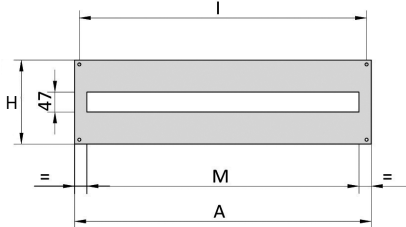
Панели/Двери для модульного оборудования OptiBox M с вырезом высотой 47 мм
