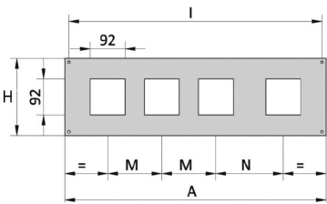
Панели/Двери модульные для измерительных приборов OptiBox M с 4 вырезами 92х92 мм
