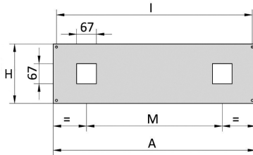
Панели/Двери модульные для измерительных приборов OptiBox M с 2 вырезами 67х67 мм
