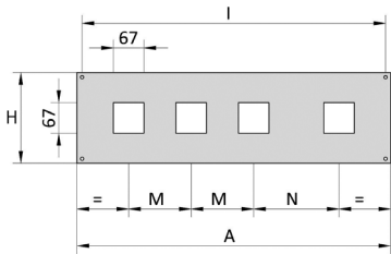
Панели/Двери модульные для измерительных приборов OptiBox M с 4 вырезами 67х67 мм
