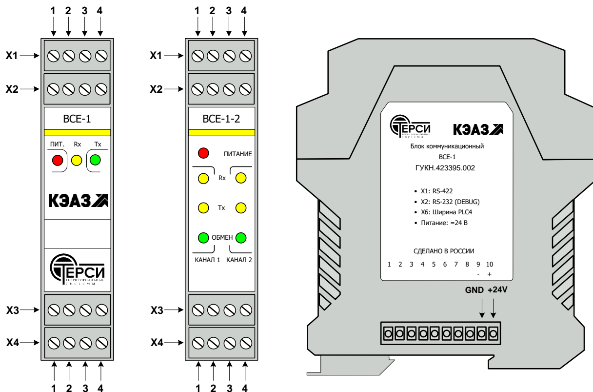
Рисунок 1 Внешний вид блока BCE-1-X и расположение разъёмов
