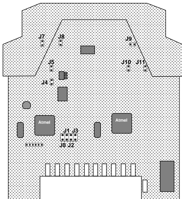
Рисунок 2 Расположение переключек на плате блока BCE-1-X
