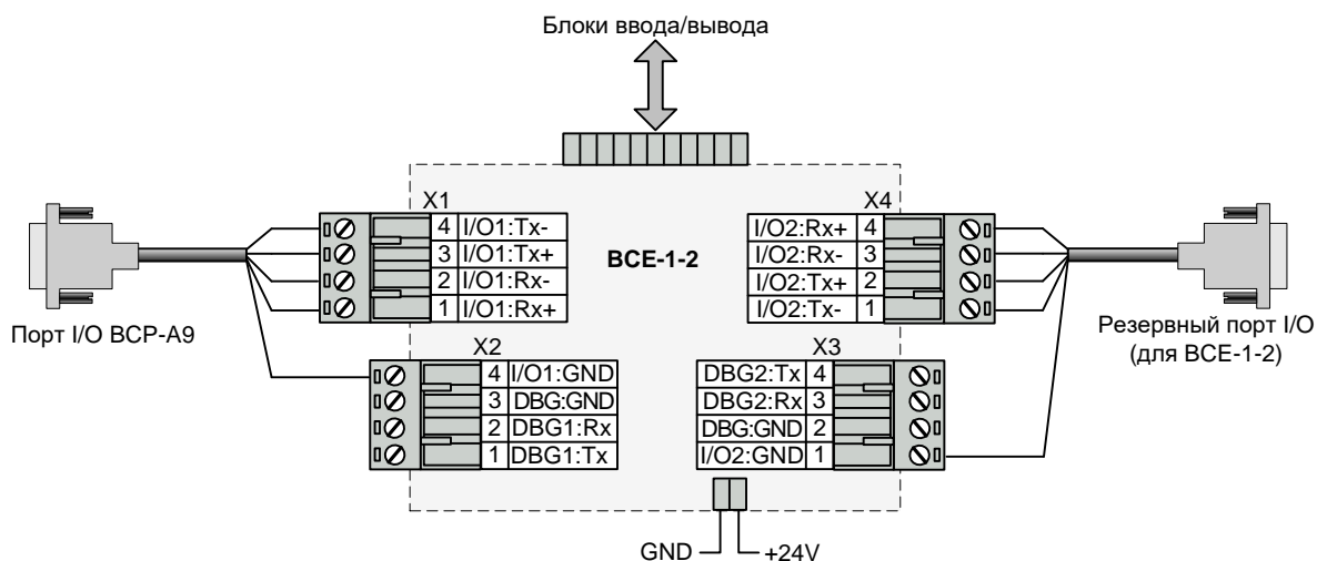
Рисунок 4 Схема подключения блока ВСЕ-1-Х
