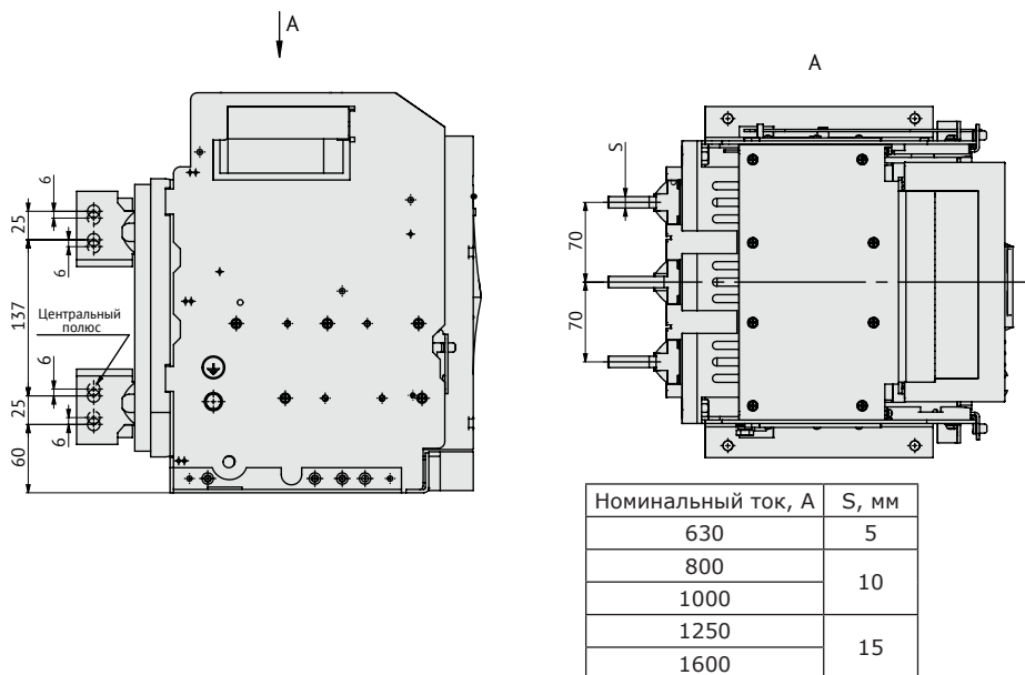
Рисунок А.7 – Автоматический выключатель OptiMat A-630-1600-S1 выдвижного исполнения на номинальные токи 630 – 1600 А с вертикальным расположением выводов
