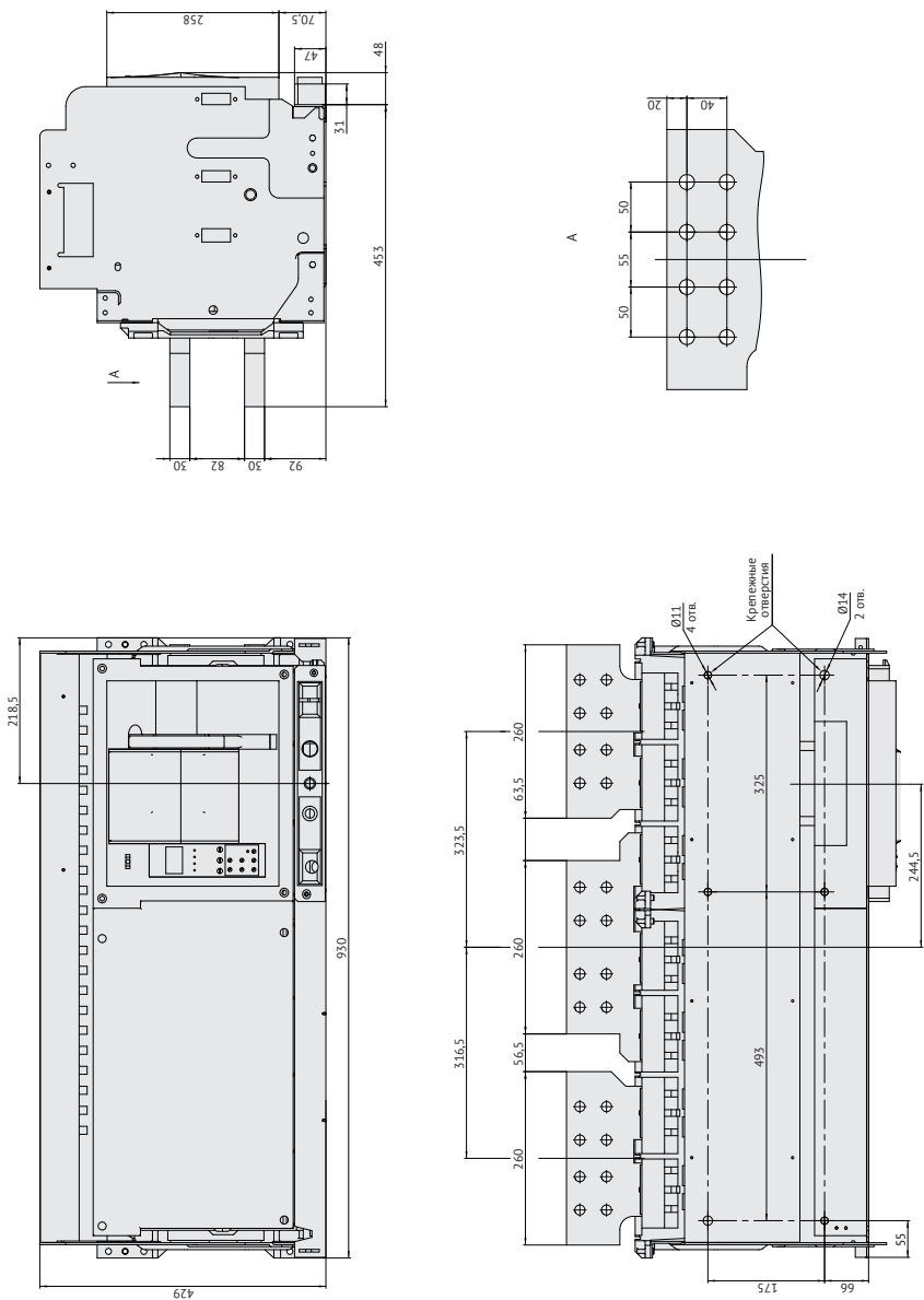
Рисунок А.10 – Автоматический выключатель OptiMat A-6300-S6 выдвижного исполнения на номинальный ток 6300 А
