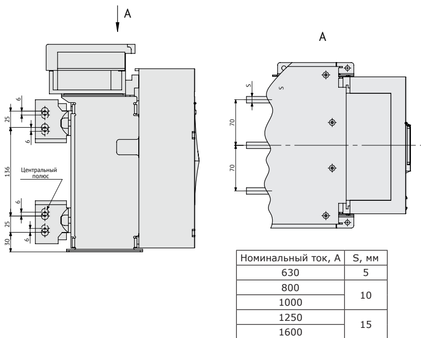
Рисунок А.3 – Автоматический выключатель OptiMat A-630-1600-S1 стационарного исполнения на номинальные токи 630 – 1600 А с вертикальным расположением выводов
