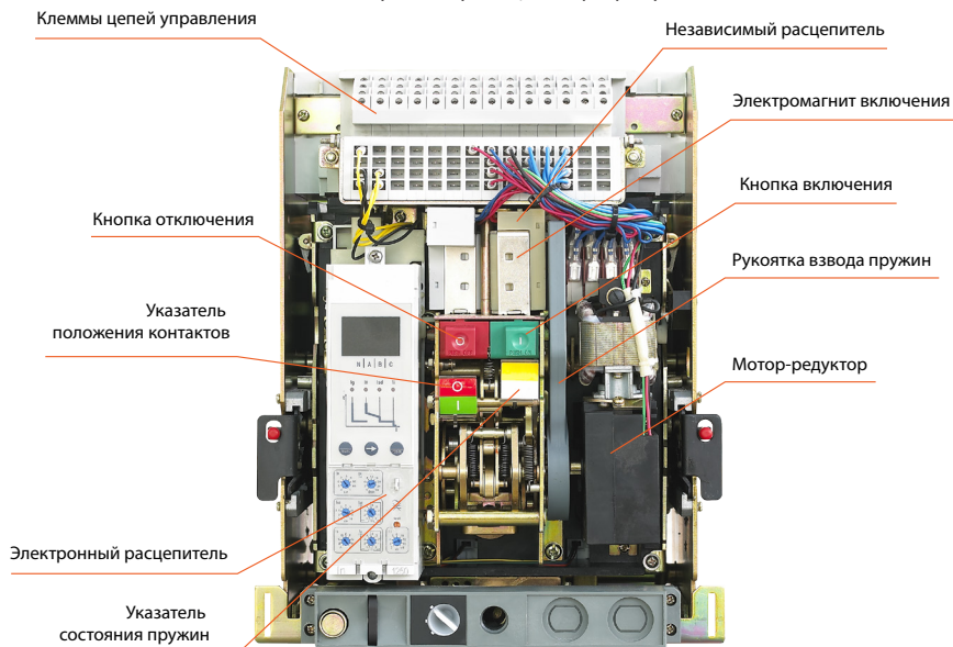
Рисунок 1 – Выключатель OptiMat A-S1
