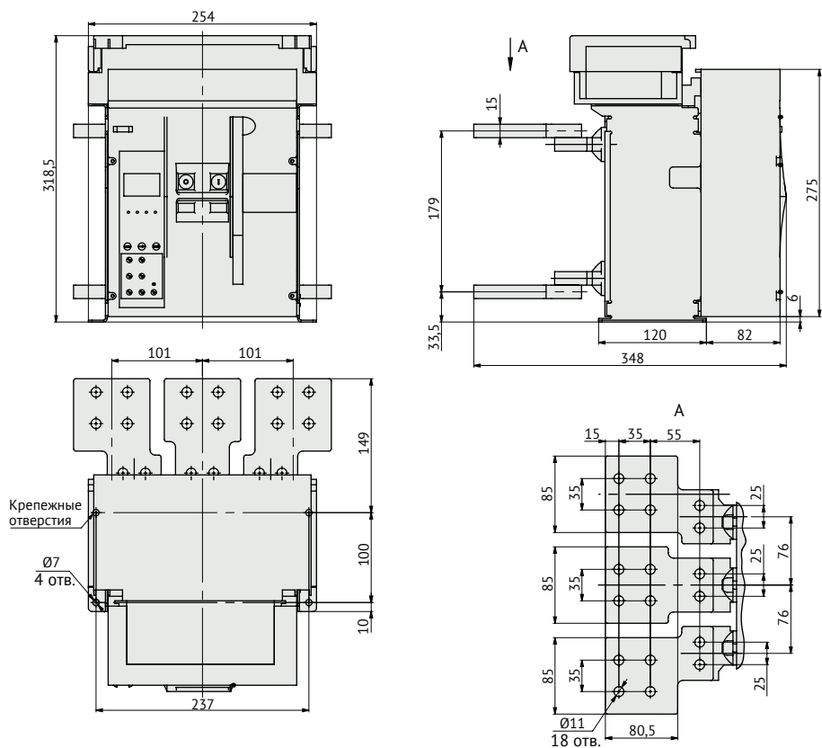
Рисунок А.2 – Автоматический выключатель OptiMat A-1600-S1 стационарного исполнения на номинальный ток 1600 А с горизонтальным расположением выводов с установленными расширителями полюсов
