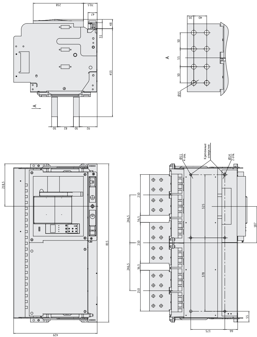
Рисунок А.9 – Автоматический выключатель OptiMat A-5000-S5 выдвигного исполнения на номинальный ток 5000 А
