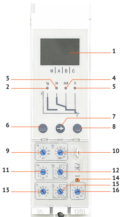
Рисунок 3 - Микропроцессорный расцепитель MR 5.0
