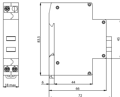
Рисунок Б.2 – Габаритные, установочные и присоединительные размеры кнопки управления типа OptiDin KM63-B
