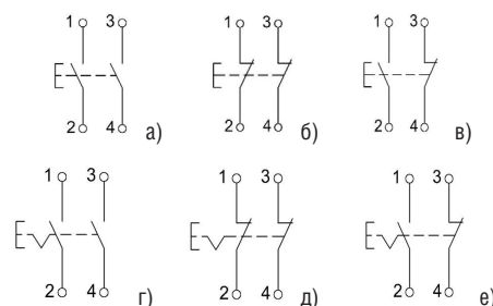
Рисунок В.1 – Принципиальные электрические схемы кнопки управления типа OptiDin KM63-A и типа OptiDin KM63-AF:
