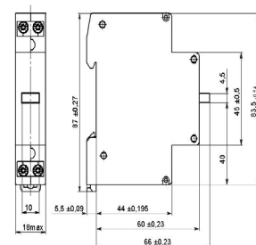
Рисунок Б.1 – Габаритные, установочные и присоединительные размеры кнопки управления типа OptiDin KM63-A и OptiDin KM63-AF
