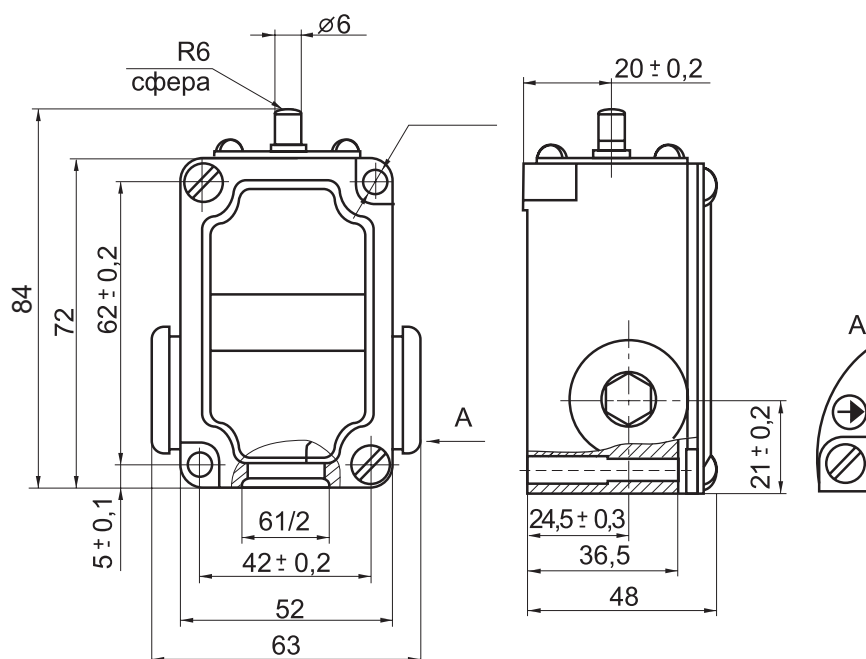
Выключатель ВПК2110
