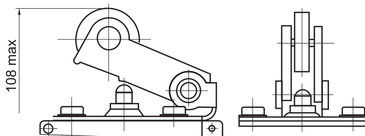
Выключатель ВПК2112
