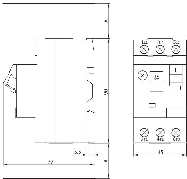
Пускатель ПРК80
