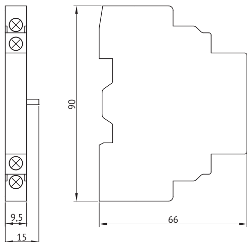
Контакт вспомогательный боковой КВБ80
