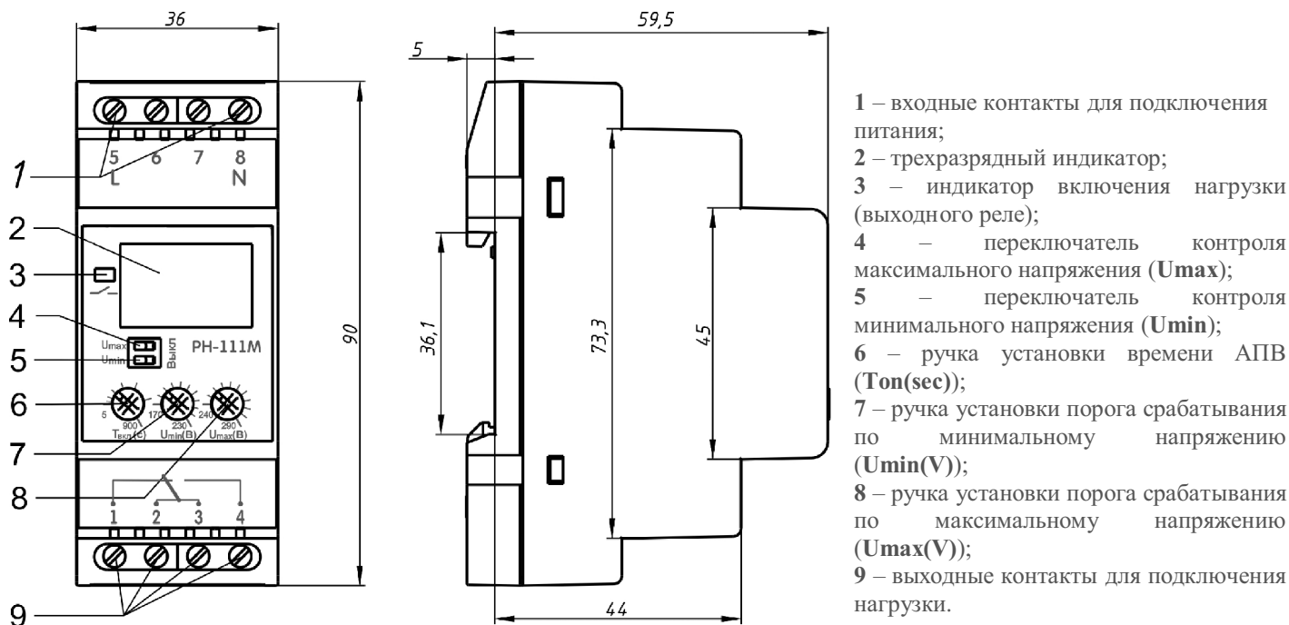
Рисунок 1 – Органы управления, габаритные и установочные размеры OptiDin PH-111M
