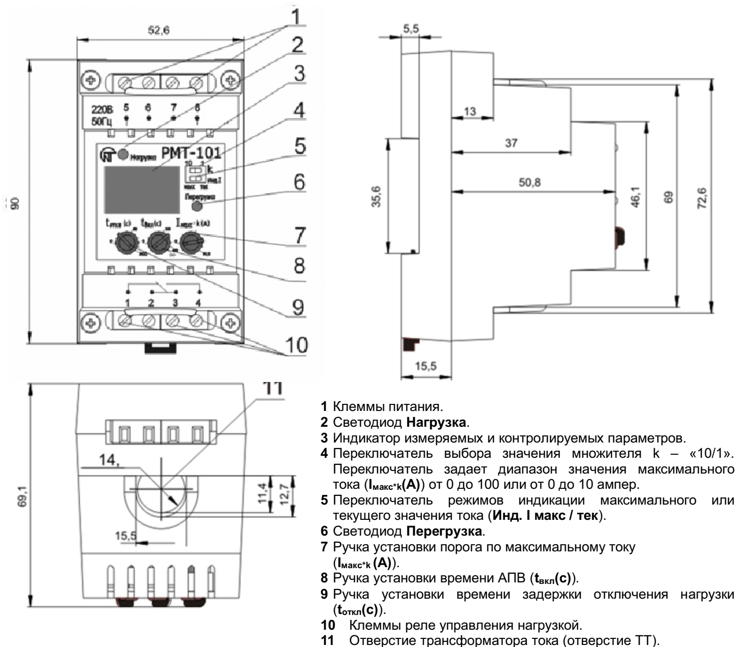
Рисунок 1 – Органы управления, габаритные и установочные размеры OptiDin PMT-101
