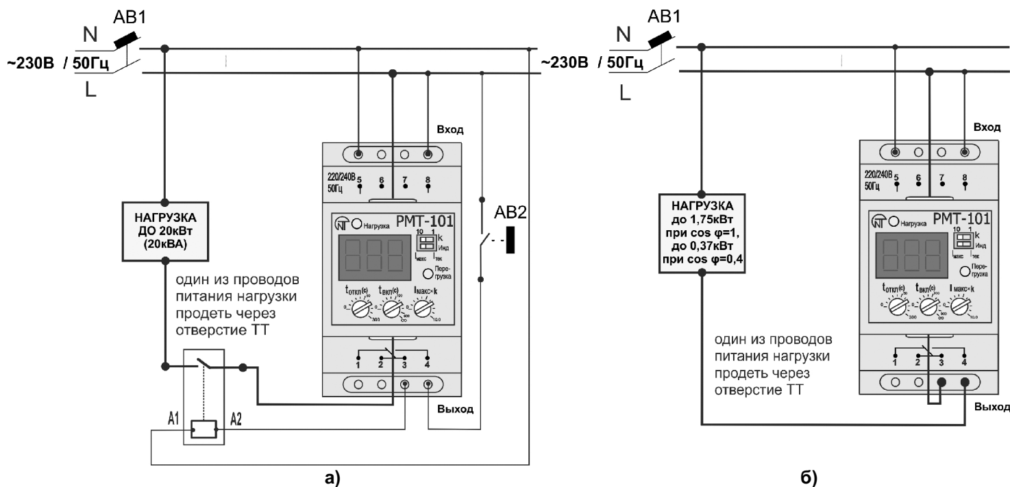
Рисунок 2 – Схема подключения OptiDin PMT-101
