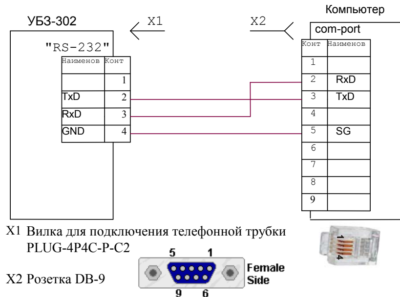
Рисунок 2.2 - Схема подключения OptiDin УБЗ-302-01 к компьютеру
