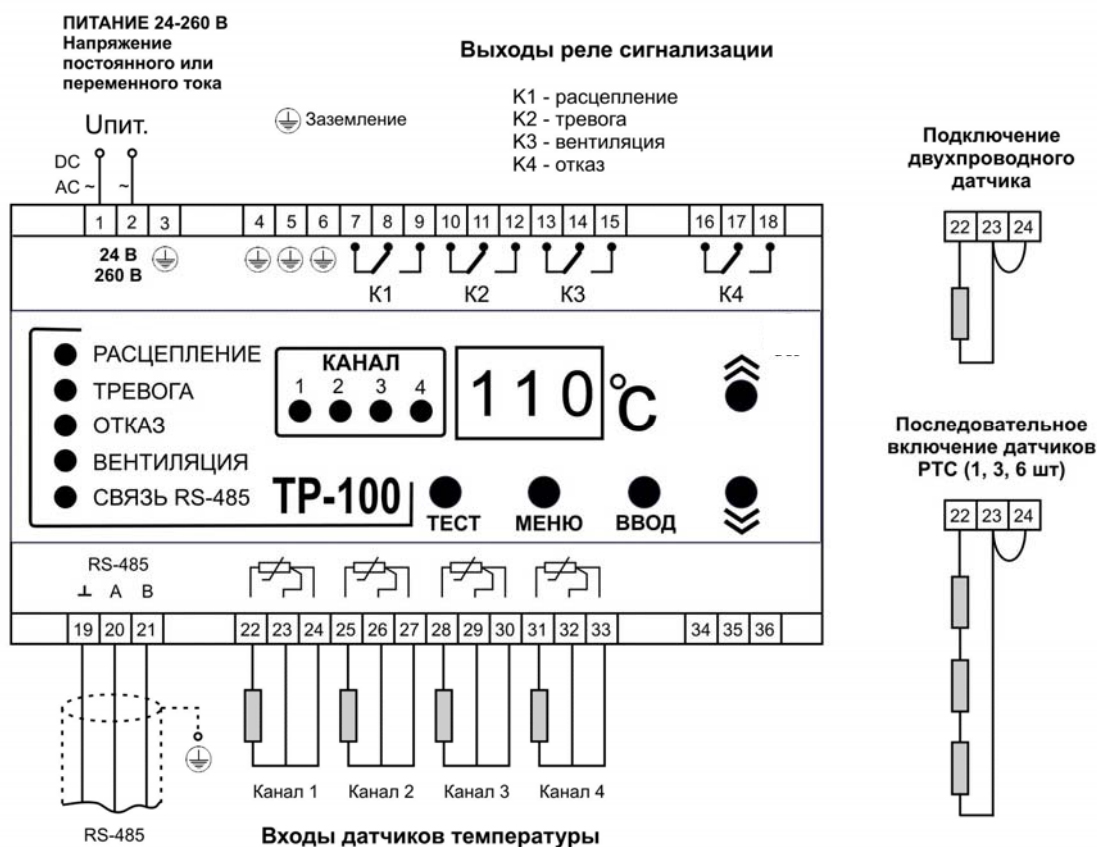
Рисунок 2 – Электрические соединения OptiDin TP-100
