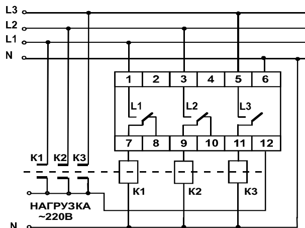
Рисунок 3 - Схема подключения OptiDin ПЭФ-301 при токе нагрузки более 16 А
