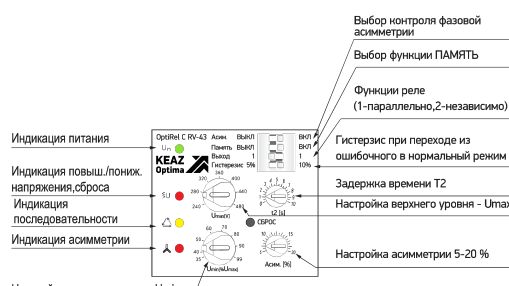
Рисунок А.2 – Вид со стороны лицевой панели реле OptiRel C RV-43
