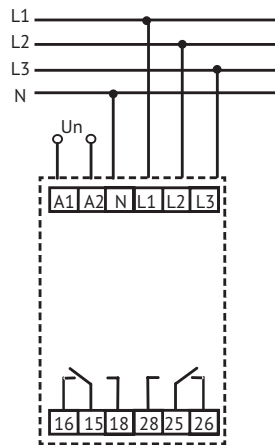
Рисунок В.1 – Схема подключения реле OptiRel C RV-43
